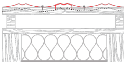
DETALJ MONTAŽE
