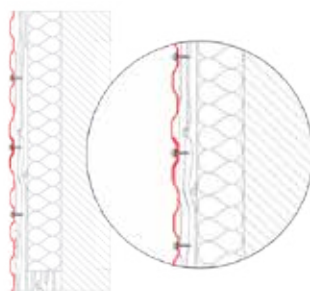
FASADNO PROFILISANJE PRESEK HORIZONTALNE MONTAŽE
